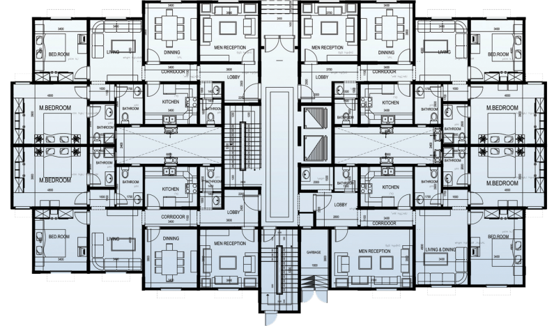
الدور الأرضي
